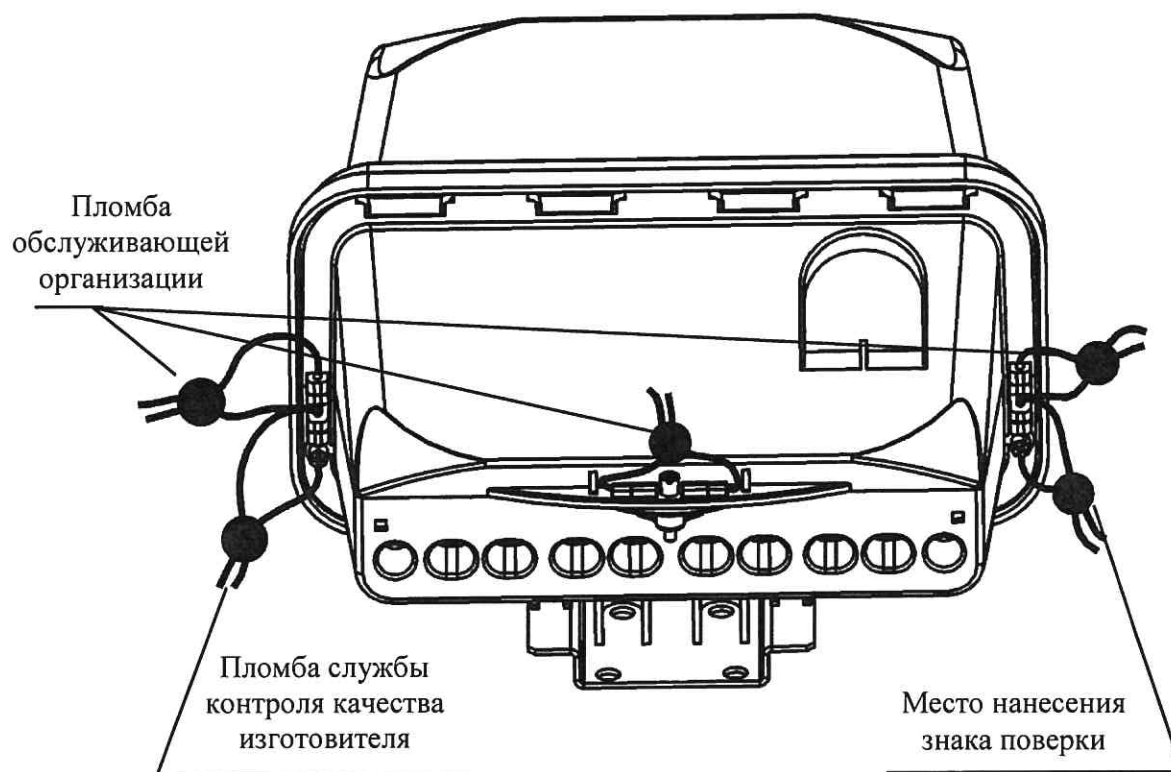
в) счетчики в корпусе SPLIT
