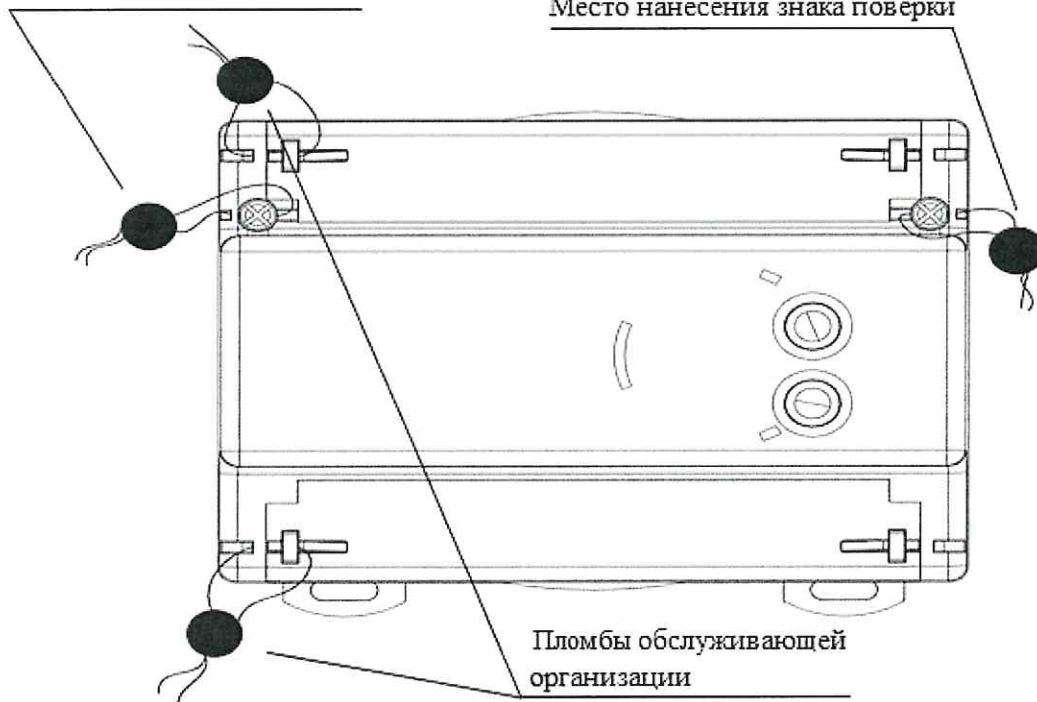
а) счетчики в корпусе 9мTH35
